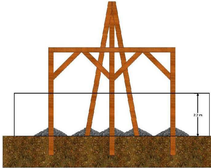
Εικόνα 10. Πρόσψη ιστού-εξέδρας-περίφραξης
