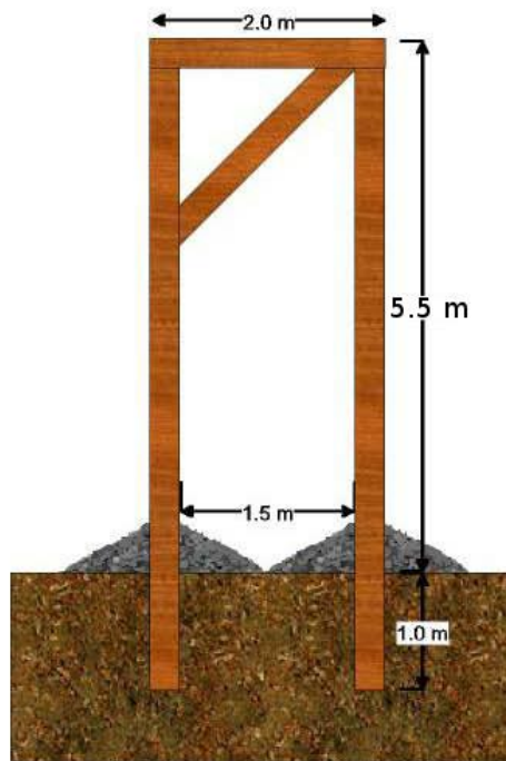
Εικόνα 8. Πλάγια όψη εξέδρας
