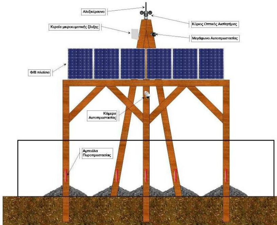
Εικόνα 11. Πρόσψη ιστού με τις συσκευές των υποσυστημάτων
