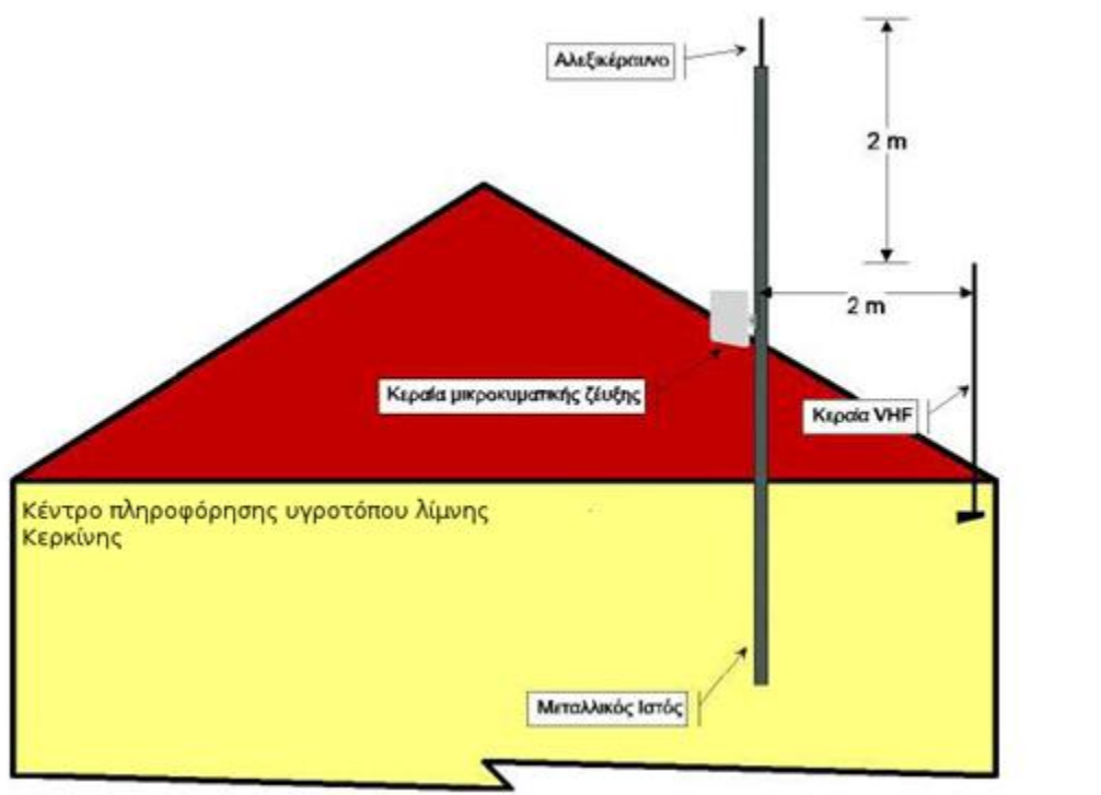
Εικόνα 16. Ο ιστός στο κτήριο που θα εγκατασταθεί το κέντρο ελέγχου στο Κέντρο πληροφόρησης υγροτόπου Κερκίνης, με τις συσκευές των υποσυστημάτων
