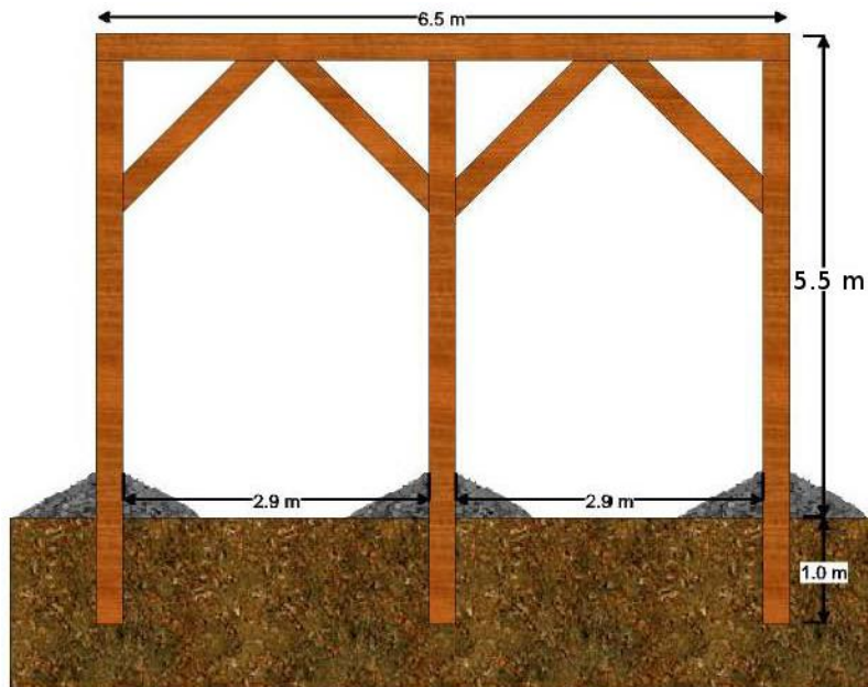
Εικόνα 6. Πρόσοψη εξέδρας
