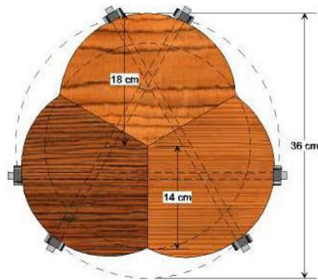
Εικόνα 4. Λεπτομέρεια σύνδεσης στύλων στην κορυφή του ιστού με ράβδους που έχουν σπείρωμα (κάτοψη)
