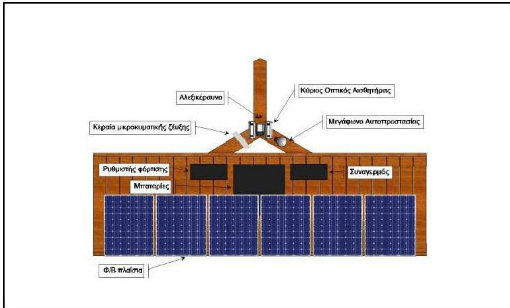
Εικόνα 12. Κάτοψη ιστού με τις συσκευές των υποσυστημάτων
