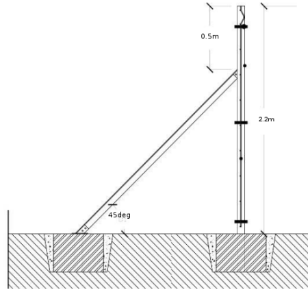
Εικόνα 15. Τομή σύνδεσης αντηρίδας με περίφραξη
